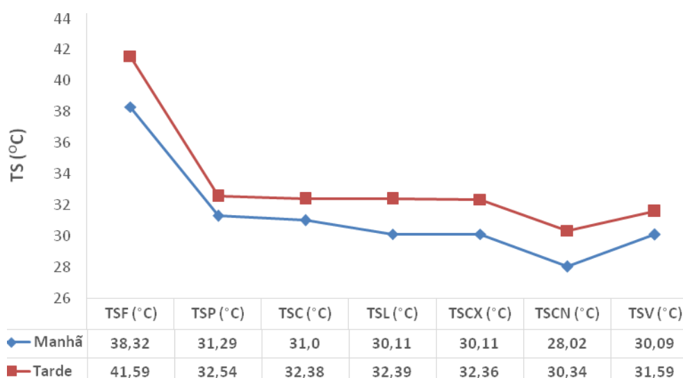
Figura 2 Temperaturas superficiais nas diferentes regiões corporais de cabritos Anglo Nubiano nos turnos manhã e tarde.
